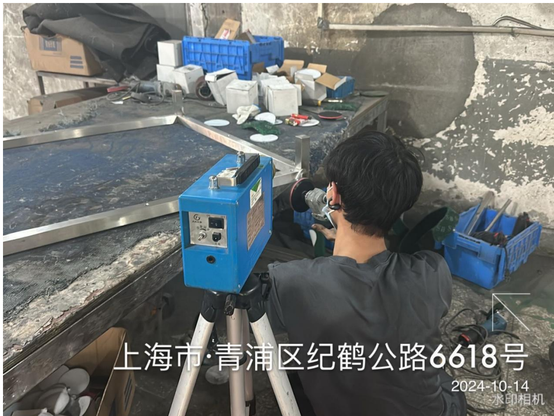
打磨操作位
